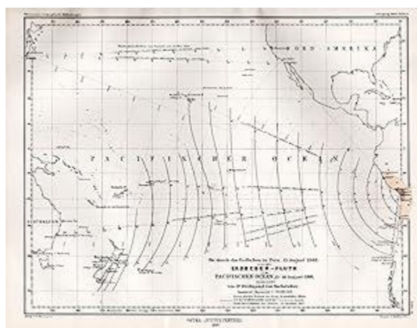
Above, from 63 Hochstetter: Die Erdbebenfluth im Pacifischen Ocean
